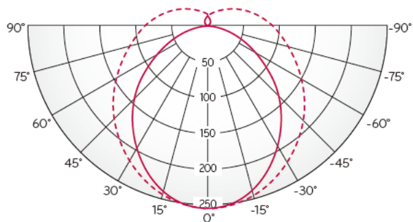
Lichtstärkeverteilung/ Luminance Intensity Distribution
